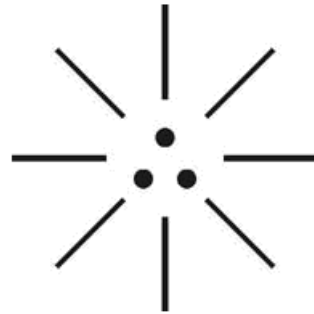
(CNO Fundamental)
