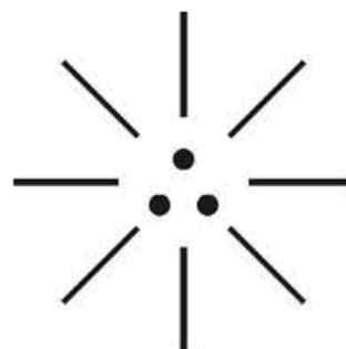
(NEUTRINOS)
