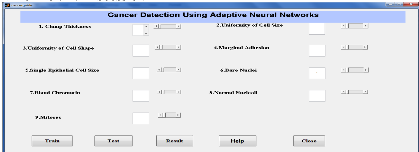
Figure4:-FRONT GUI
